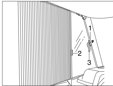
Fig. 87 Tendina oscurante pieghevole del finestrino del conducente e del passeggero
